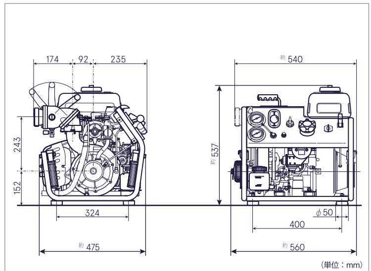
外観図
