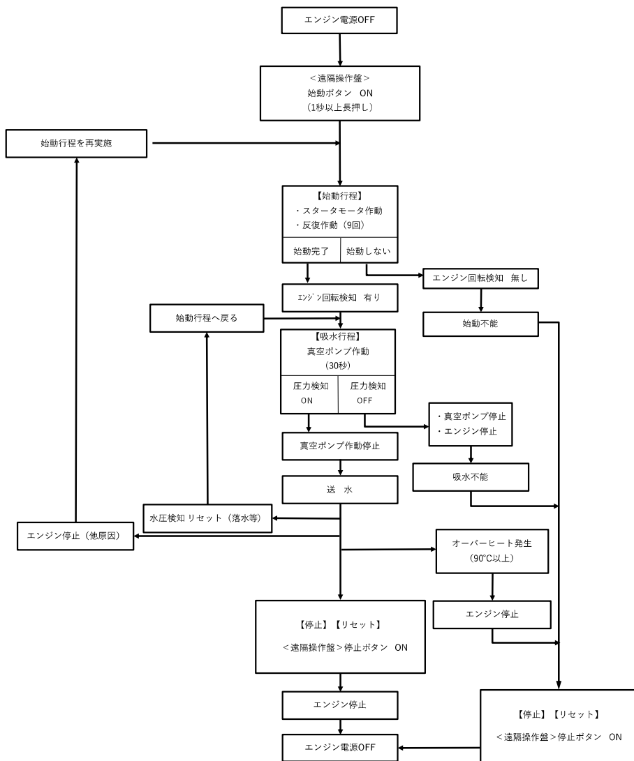
■遠隔操作盤による自動運転モード作動系統図
