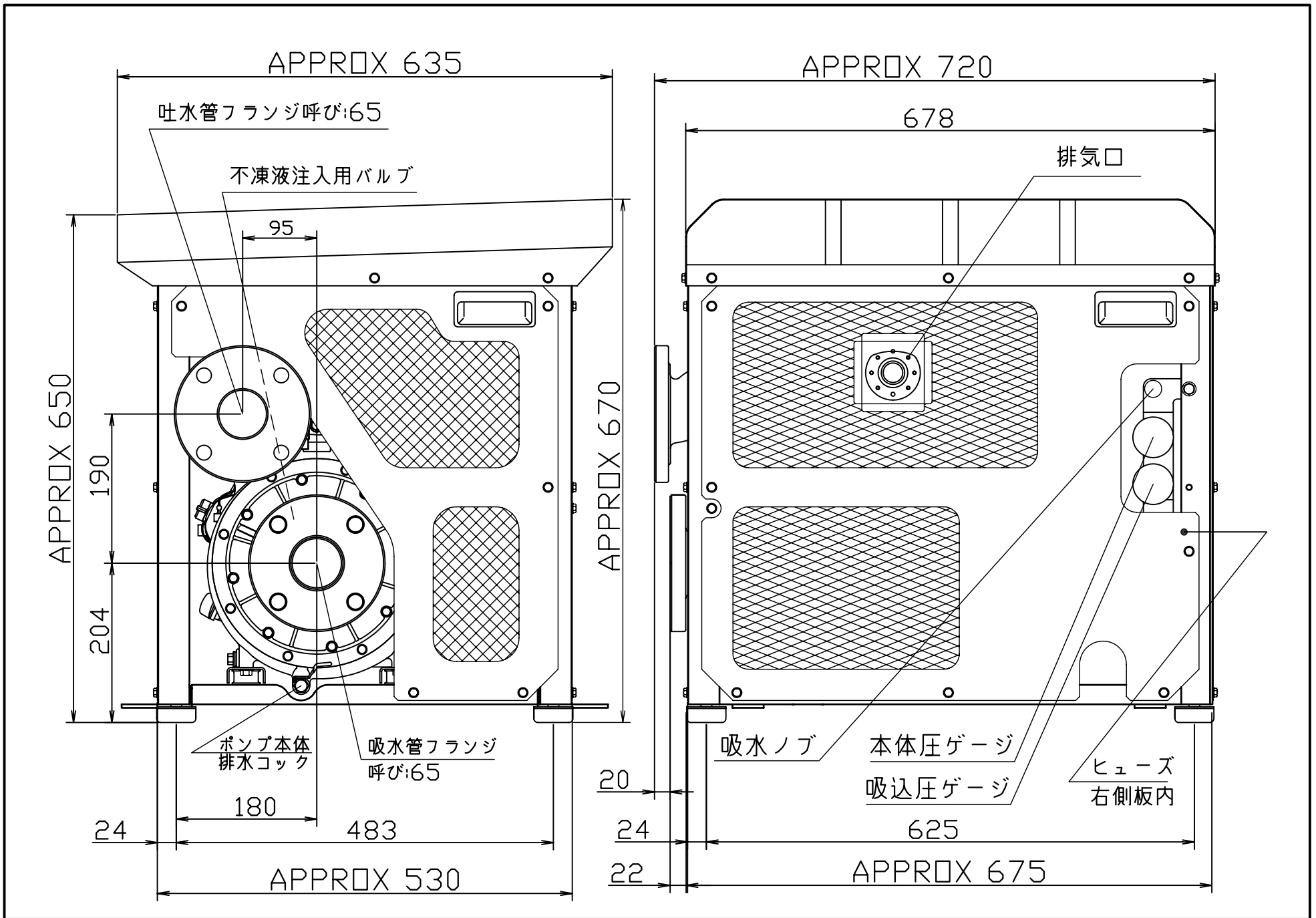
LG450AM 外観図
