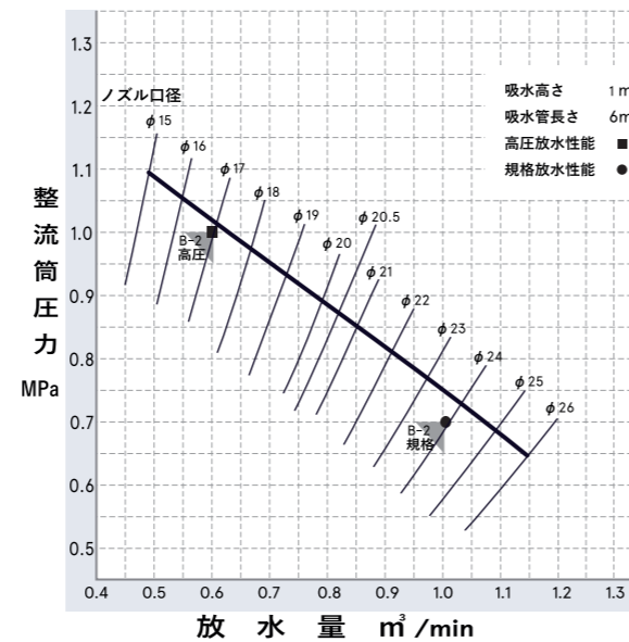
ポンプ性能曲線
