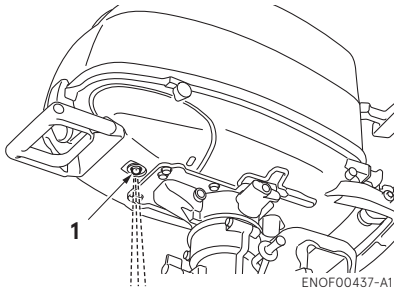
1. Orifice de contrôle de l'eau de refroidissement
