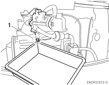
1. Vis de vidange du carburateur
