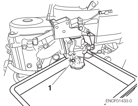
1. Vergaserablassschraube
